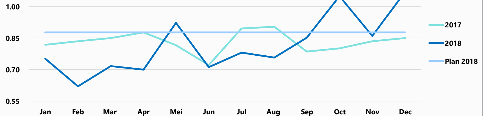
Volume Bulanan Produksi Batubara (juta ton)
