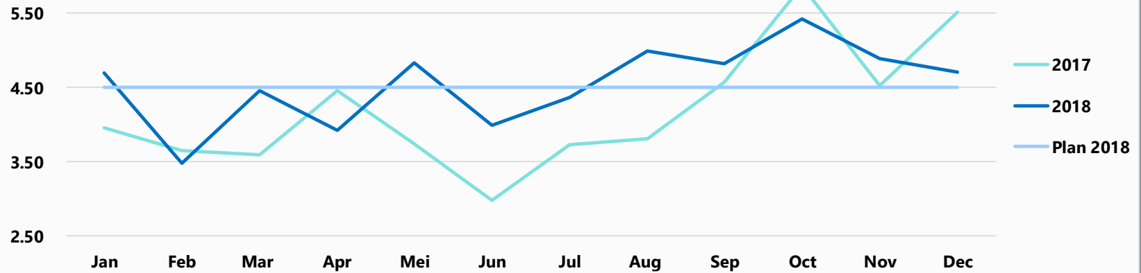
Volume Bulanan Batuan Penutup (juta bcm)
